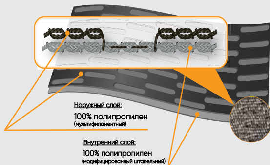
ЯЧЕЙСТОЕ ДВУХСЛОЙНОЕ ПОЛОТНО ПАТЕНТ RU 165 334
